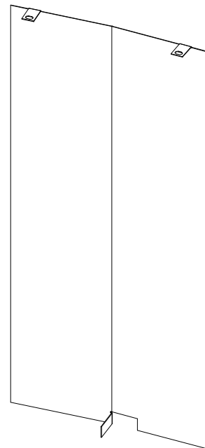
Strahlenschutzblech Heat protection panel Panneau de protection thermique Bescherming tegen hitte panel
