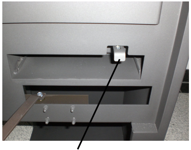
Bedienhebel für den Feuerrost
