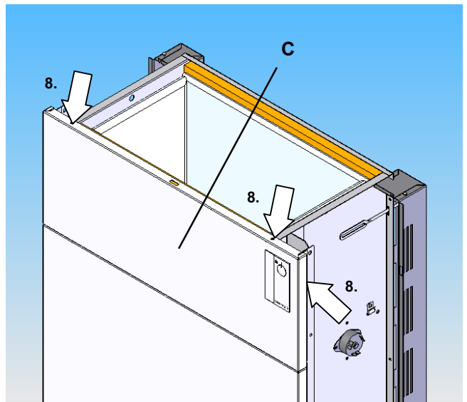
fig.4 Enlevez la paroi frontale supérieure
