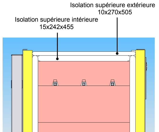
fig.7 Isolations supérieures
