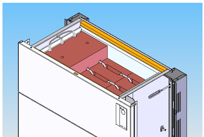
fig.6 Résistances et briques de couverture
